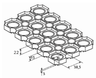
Схема изделия
