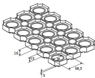
Схема изделия
