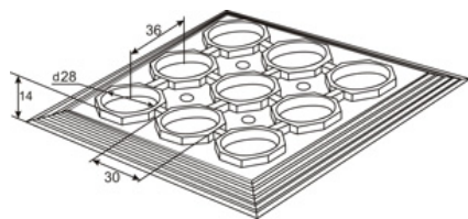
Схема изделия
