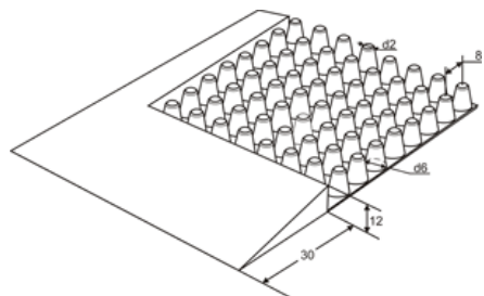
Схема изделия
