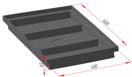
Схема изделия
